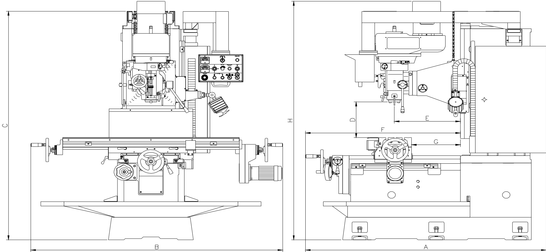
TMB-8PS/MV/IV 外型尺寸圖
