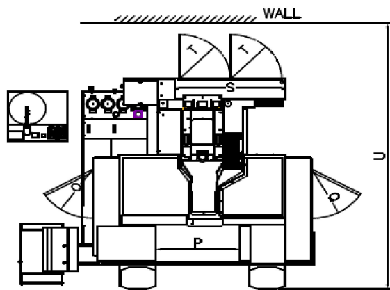
TMQ-8外型尺寸圖
